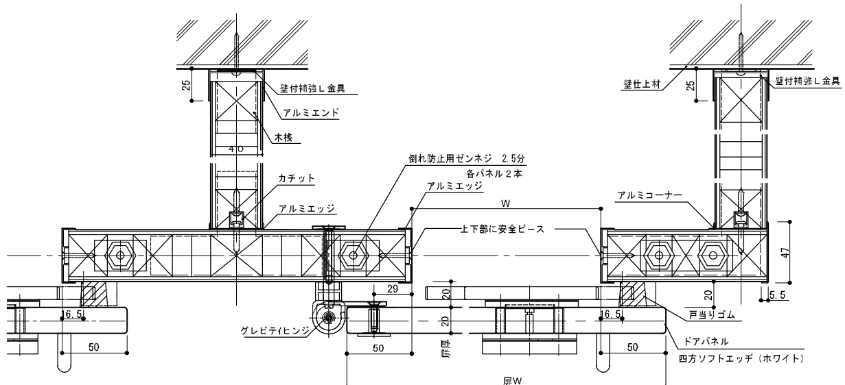
幼児用ブース平面図 (原付)
