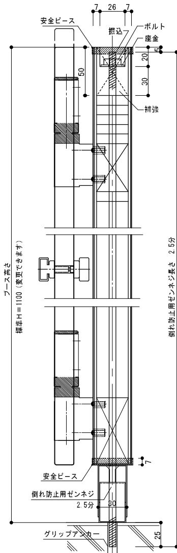
パネル補強縦断面図 (コンクリート下地)
