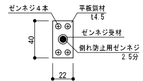
ゼンネジ受けベースプレート図
