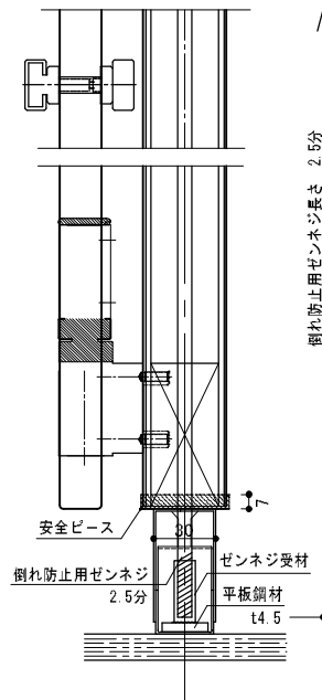
パネル補強縦断面図 (上床下地)
